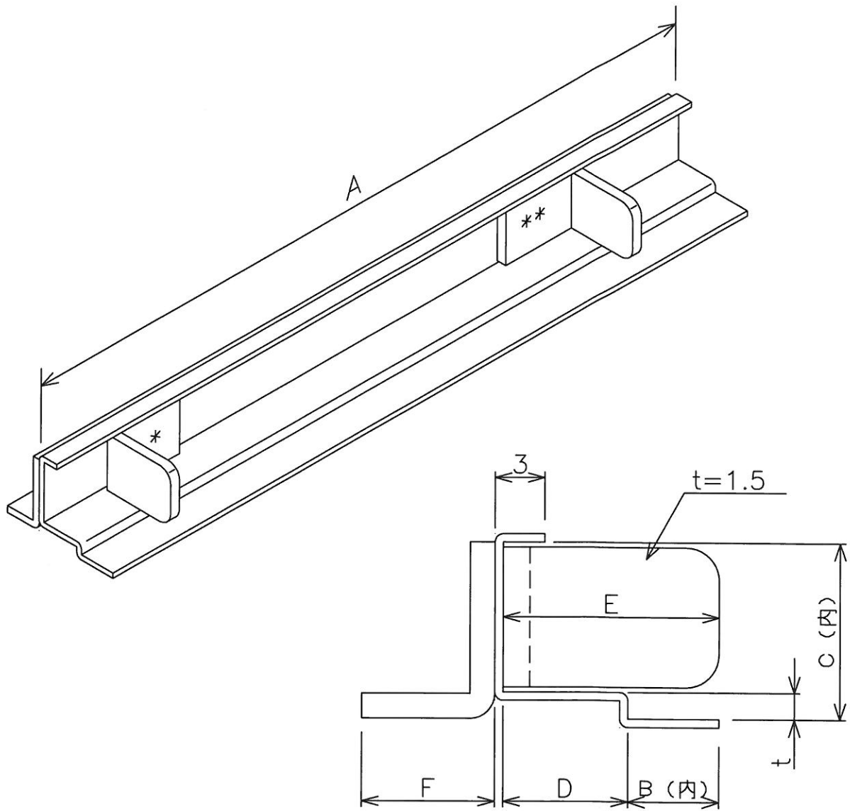
側面詳細図
