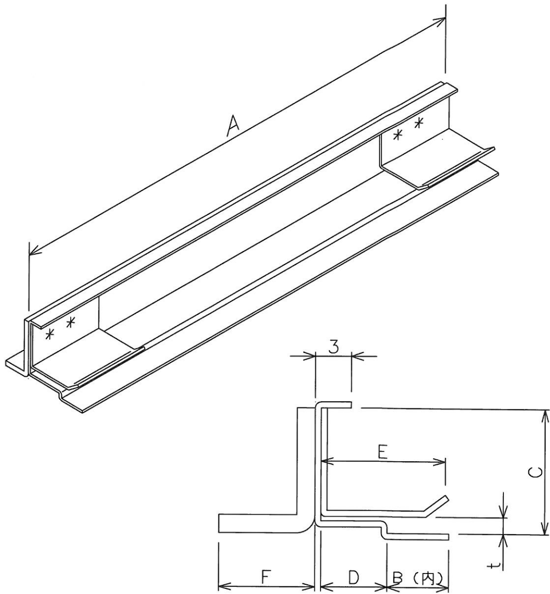
側面詳細図
