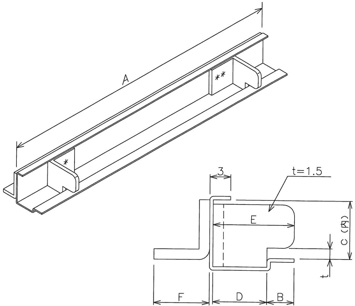
側面詳細図
