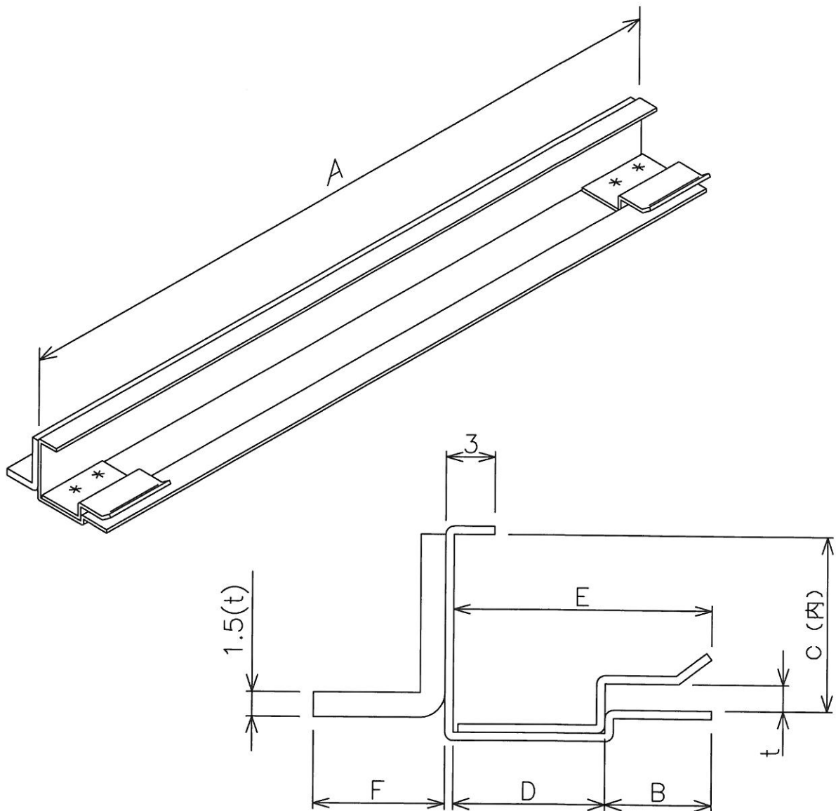
側面詳細図
