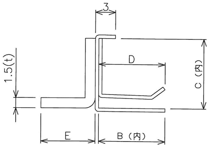
側面詳細図
